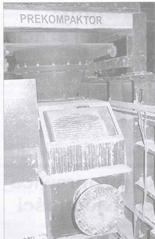
Zgniatacz (kompaktor) – serce nagrodzonej linii technologicznej
