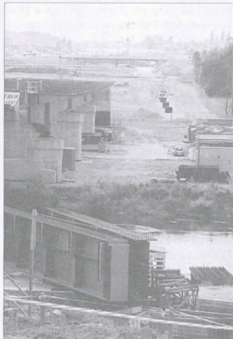
Końcowe prace przy budowie przepustu długości ok. 60 m dla Strumienia Junikowskiego, krzyżujące się w tym miejscu z autostradą. Po ich zakończeniu, koryto strumienia zostanie przesunięte w kierunku zachodnim o ok. 20 m. W dalszym planie widoczna jest kotłownia SM „Lubonianka” przy ul. Źródlanej.
