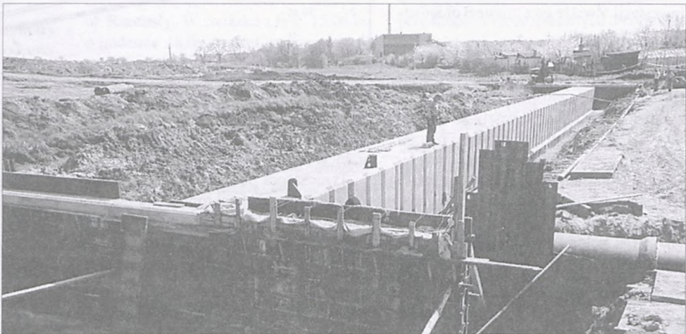
Końcowe prace przy budowie przepustu długości ok. 60 m dla Strumienia Junikowskiego, krzyżujące się w tym miejscu z autostradą. Po ich zakończeniu, koryto strumienia zostanie przesunięte w kierunku zachodnim o ok. 20 m. W dalszym planie widoczna jest kotłownia SM „Lubonianka” przy ul. Źródlanej.
