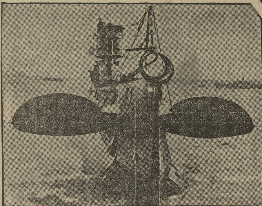
NOWA ŁÓDź PODWODNA Na rycinie widzimy nową amerykańską łódź podwodną zaopatrzoną w pletwy zapewniające większe bezpieczeństwo w nurkowaniu.
