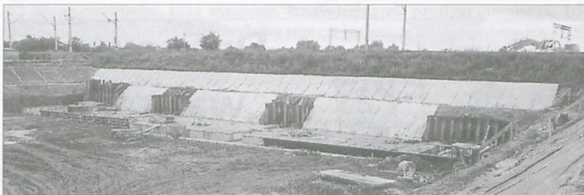
Zdj. 5. Wiadukt kolejowy WK5 - fundamenty wschodniego wylotu tunelu
