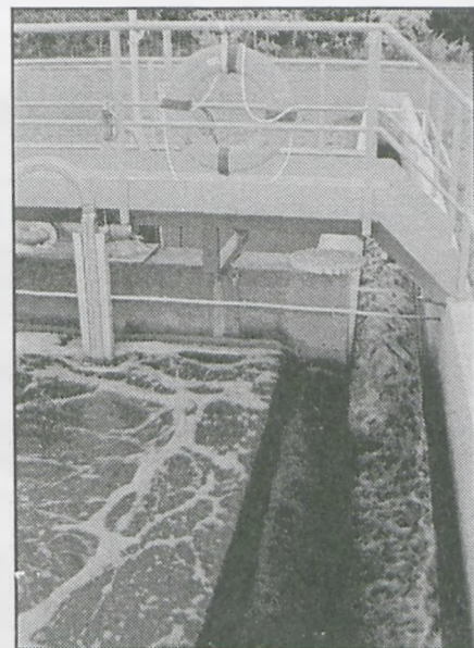
Reaktor biologiczny — napowietrzanie ścieków
