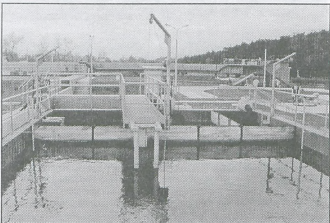
Reaktor biologiczny (ujęcie z drugiej strony)
