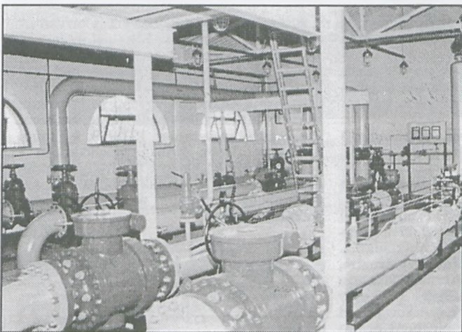
Urządzenia nowej stacji redukcji gazu
