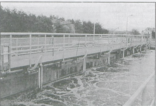
Reaktor biologiczny — napowietrzanie ścieków
