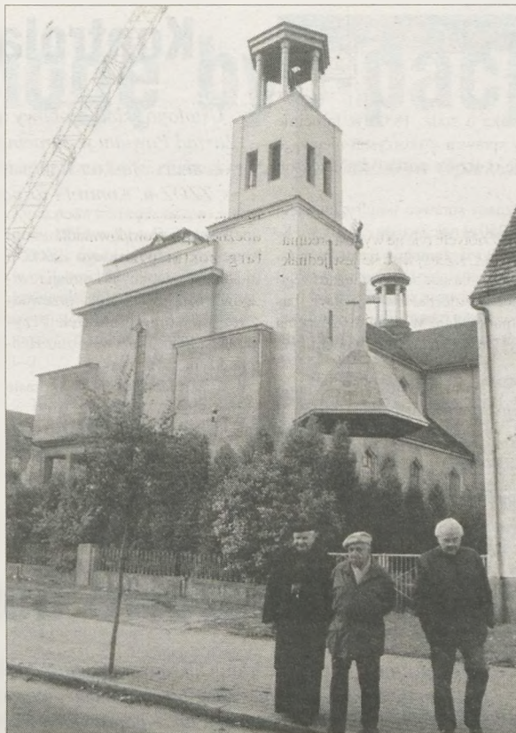
Montaż elementów wieży obserwowali proboszcz parafii Chrystusa Króla ks. prałat Stanisław Adamski, autor projektu rchitektonicznego wieży Stanisław Koziełski i wykonawca projektu konstrukcyjnego Roman Neyder
