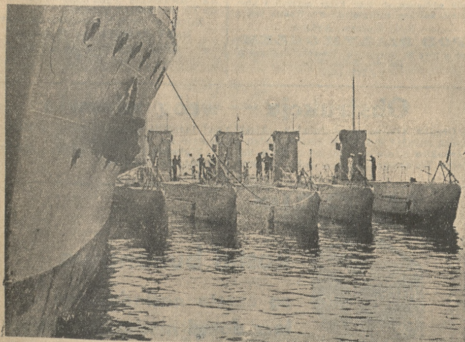
Flotyla łodzi podwodnych „Weddingen” składa się z nurkowców nowego typu o wyporności 750 tonn, które w promieniu działania i w uzbrojeniu przewyższają łodzie starszego typu o wyporności 1 000 tonn.
