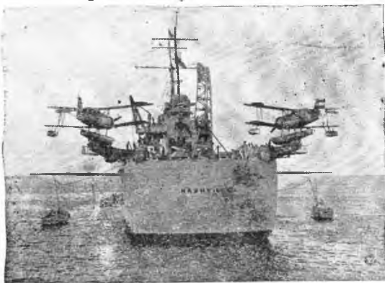
Potężny amerykański krążownik-lotniskowiec „Nashville” w czasie ćwiczeń na wodach amerykańskich. Na pokładzie widoczne wodnopłatawce, ustawione na swoich katapultach, gotowe w każdej chwili lotu.
