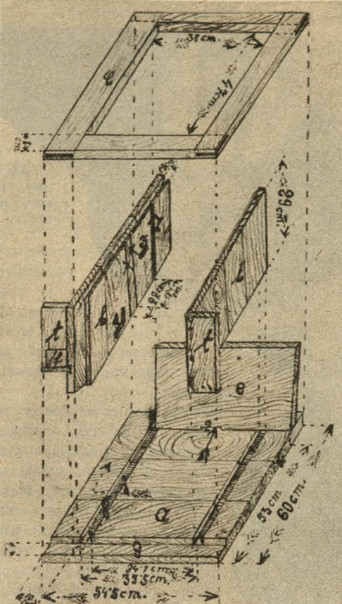
Rys. 1. Rozłożony szkielet „Ula Pom.“ a) dno b) ściany wewnętrzne c) ściana przednia e) obramowanie. 1) wylot główny 2) wylot rezerwowi. Ściany boczne i dno są wsadzone na klej.
