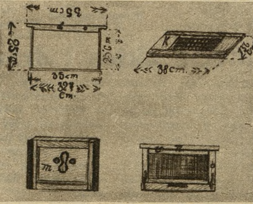
Rys. 3. Części składowe „U. P.“ Ramka, kratka, deska przegrodowa i wylot (okienko).
