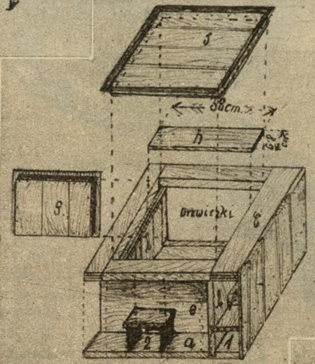
Rys. 2. Korpus ula. Obita lewa ściana. Przednia i prawa ściana nieobita 1) kanał wylotu głównego 2) bramka wylotu rezerwowego 9) drzwiczki h) powala (7 deseczek na całą powalę) j) wieko.
