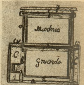
Rys. 6. Poprzeczny przekrój „U. P.“ a) dno b) ściany wewnętrzne c) przestrzeń wypchana plewami i obramowania gniazda d) ramki e) deseczki (powala) f) nadstawka g) wieko h) podkarmiaczka i) wylot główny j) wylot rezerwowi.
