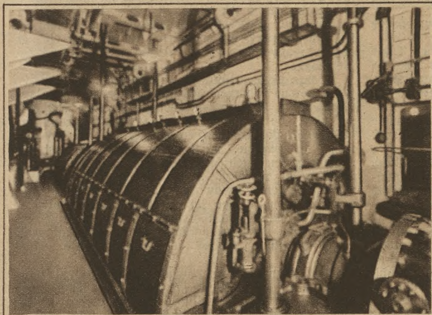
Rzut oka w halę maszyn okrętowych. Olbrzymia turbina morska
